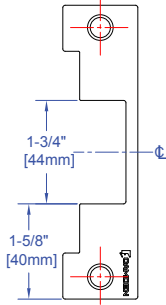
CX-EMP100: 'ANSI' carré-cadre de porte en métal, applications de ligne centrale. Compatible avec tous les ensembles de serrures cylindriques.
