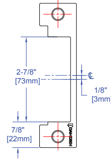
CX-EMP310: 'ANSI' carré-cadre en métal, pêne dormant utilisé uniquement pour la fonction de verrouillage nocturne. Compatible avec les ensembles de serrures Sargent-7700/ 8100, Yale 8700.
