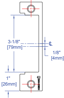
CX-EMP210: 'ANSI' carré-cadre en métal, pêne anti-retour positionné en dessous du pêne dormant. Compatible avec les ensembles de serrures Corbin Russwin, Best-45/47, Falcon, Sargent-7800/ 8200/ 9200.
