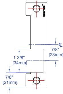
CX-EMP200: 'ANSI' carré-cadre de porte en métal, pêne anti-retour positionné au-dessus du pêne dormant. Compatible avec les ensembles de serrures Baldwin, PDQ, Marks.
