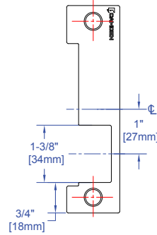
CX-EMP300: 'ANSI' carré-cadre en métal, pêne anti-retour positionné au-dessus du pêne dormant. Compatible avec les ensembles de serrures Sargent-8100/7700, Schlage, Yale 8700.
