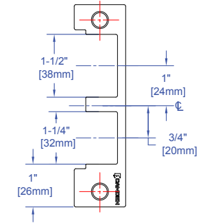
CX-EMP410: 'ANSI' carré-cadre en métal, utilisé pour un pêne dormant de 1" et pas de loquet. Compatible avec les ensembles de serrures Marks, Baldwin, Arrow, PDQ, Omnia.
