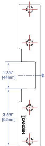
CX-EMP100W: Cadres en bois, pêne dormant utilisé uniquement pour la fonction de verrouillage nocturne. Compatible avec les ensembles de serrures Marks, Omnia, PDQ, Arrow, Accurate.
