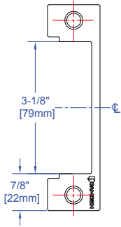
CX-EMP110: 'ANSI' carré-cadre en métal, pêne dormant utilisé uniquement pour la fonction de verrouillage nocturne. Compatible avec les ensembles de serrures Marks, Omnia, PDQ, Arrow, Accurate.
