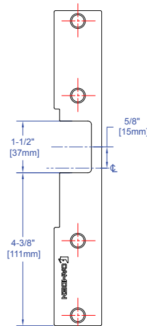
CX-EMP400W: Cadres en bois, pêne anti-retour positionné au-dessus du pêne dormant. Compatible avec tous les ensembles de serrures cylindriques.
