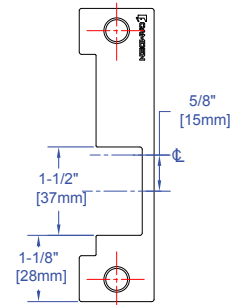
CX-EMP400: 'ANSI' carré-cadre en métal, pêne anti-retour positionné en dessous du pêne dormant. Compatible avec les ensembles de serrures Corbin Russwin, Falcon, Sargent/7800.
