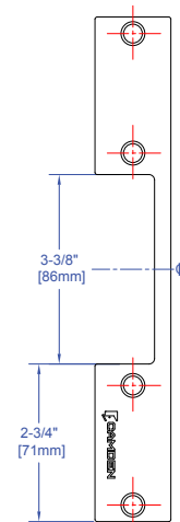
CX-EMP110W: Cadres en bois, applications de ligne centrale. Compatible avec tous les ensembles de serrures cylindriques.
