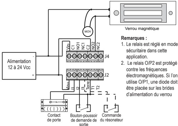
SCHÉMA DE CÂBLAGE DES MODES 1 ET 2
